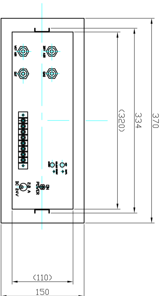
背面図
